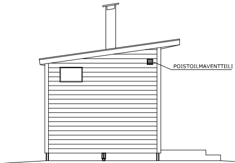
Julkisivu JS3
