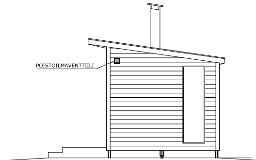
Julkisivu JS2
