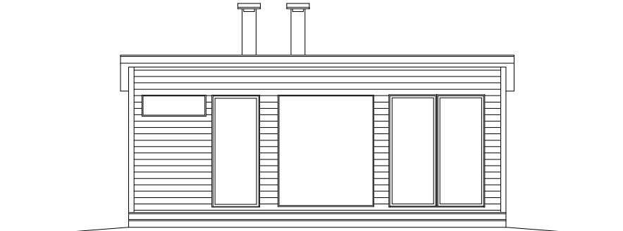
Julkisivu JS4
